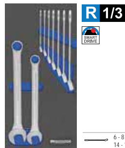
■ Set of Combination Spanners DIN 3113 A, 9 pcs
